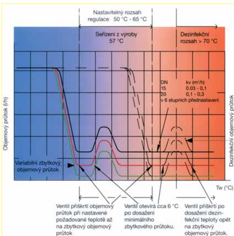
Funkčná schéma a okruhy činnosti „Aquastromu VT“ v prevádzkovej činnosti a v dezinfekčnej fáze
