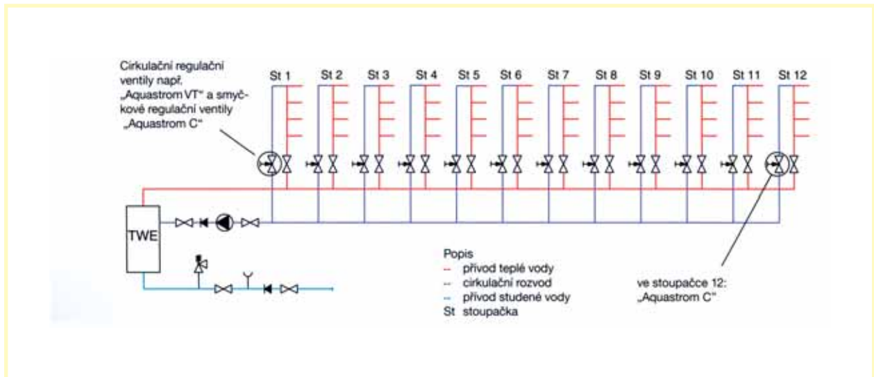
Schéma slučkového cirkulačného rozvodu teplej pitnej vody s regulačnými armatúrami „Aquistrom VT“ a „Aquistrom C“.
